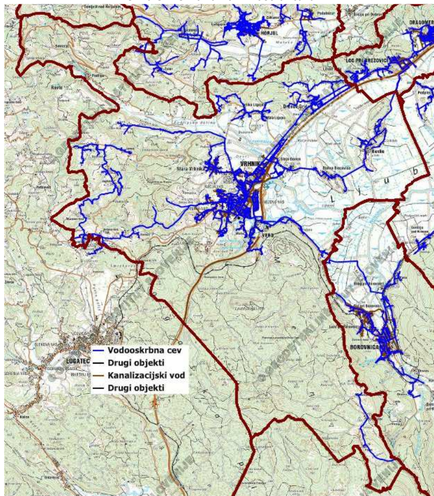
Slika 3: Komunalna infrastruktura
