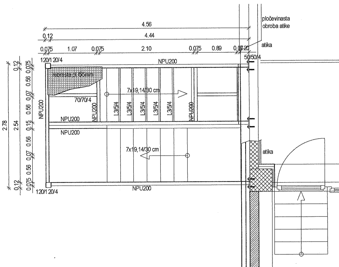
tloris 2. nadstropja
