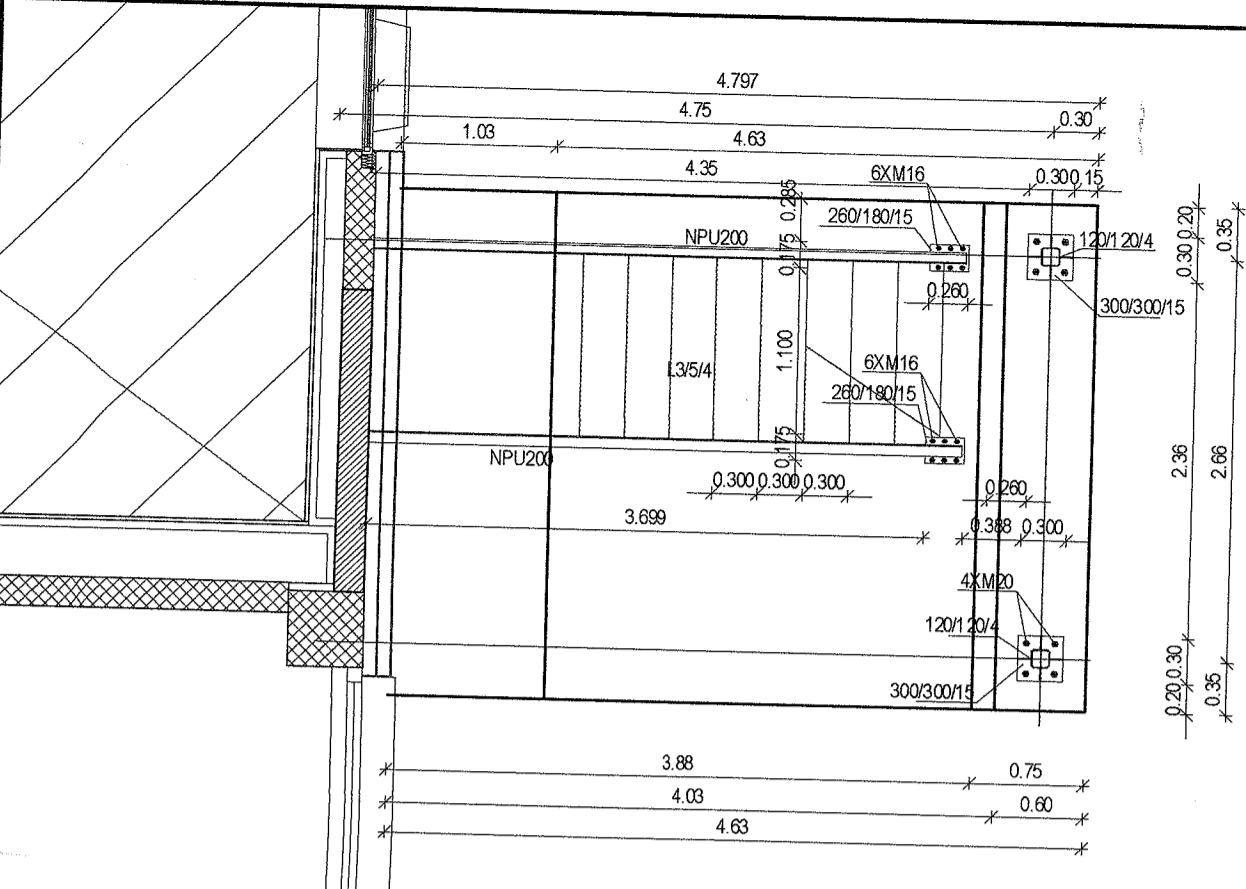
tloris temeljev
