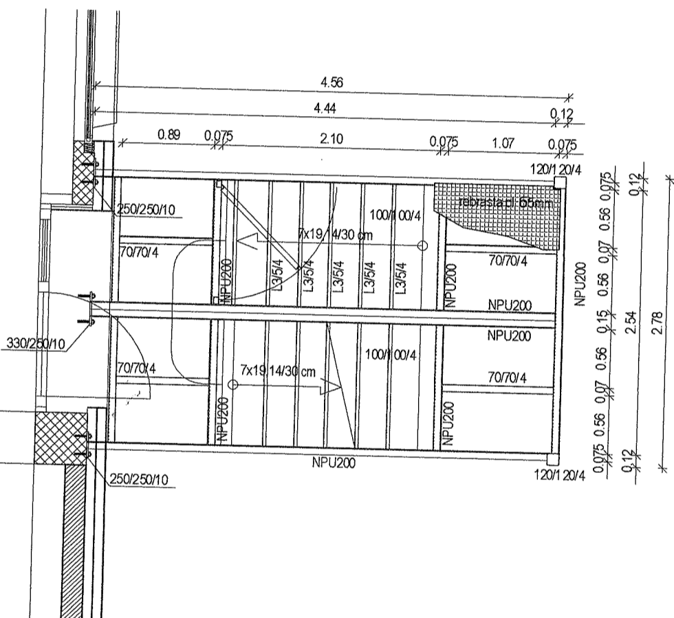
tloris 1. nadstropja
