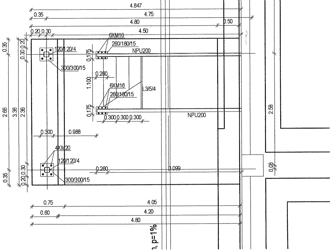
tloris temeljev
