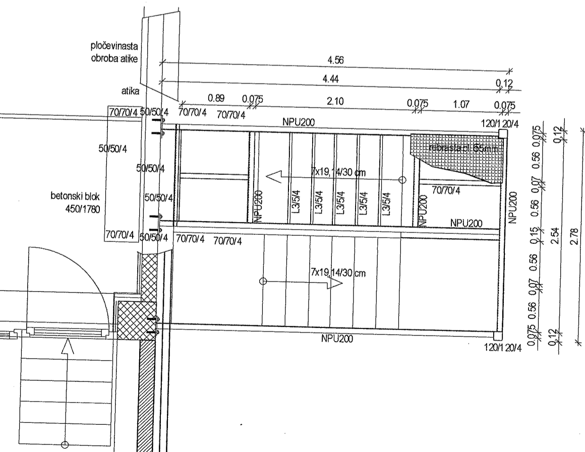
tloris 2. nadstropja
