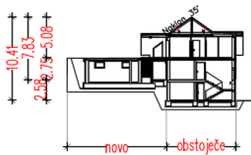
PREČNI PREREZ:
